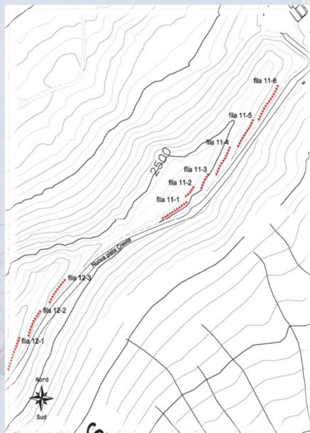
Ski area "Cresta" - Planimetria di tracciamento
