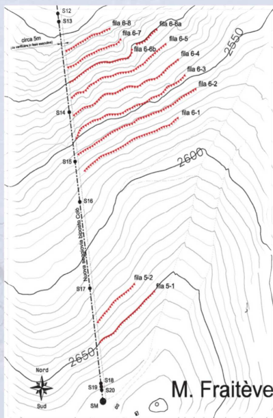
Seggiovìa "Colò" - Planimetria di tracciamento
