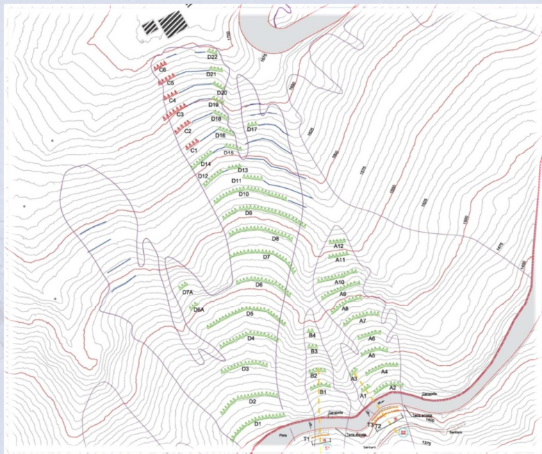
Planimetria di tracciamento
